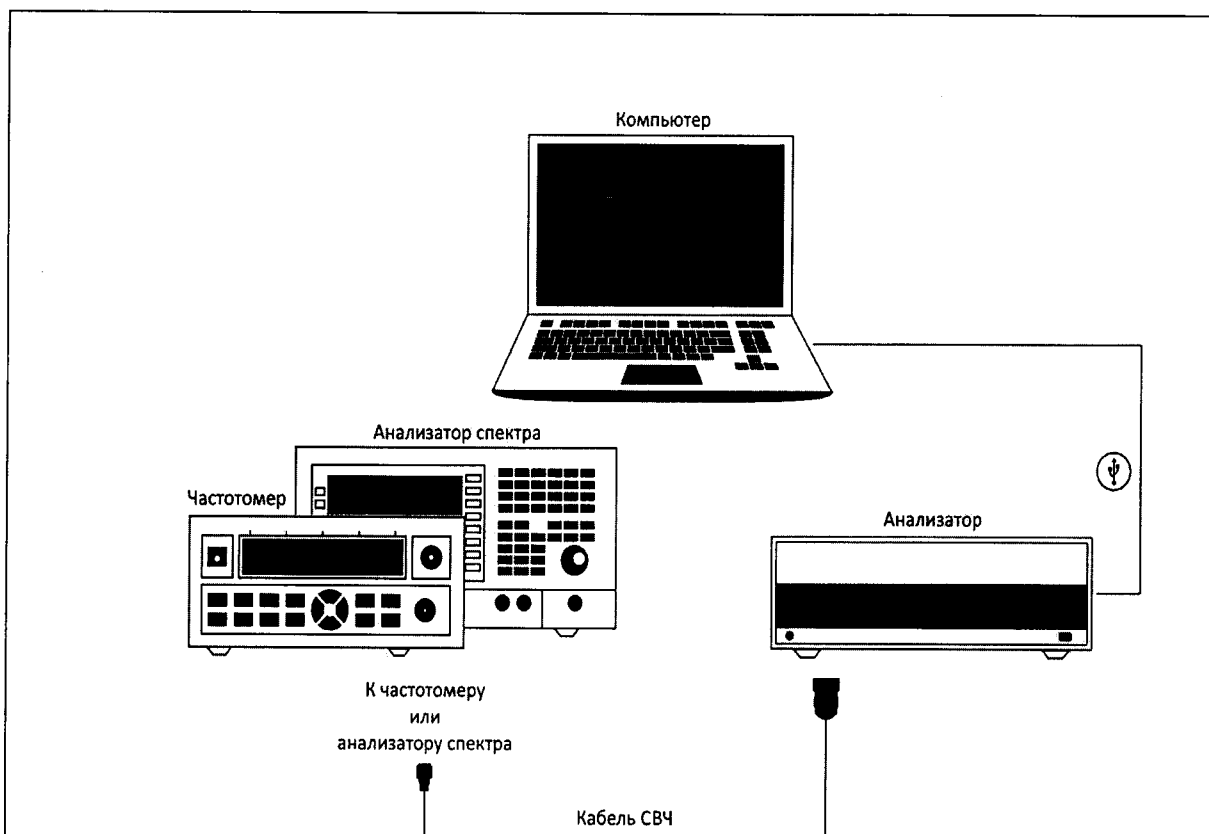
Рисунок А.3 – Схема измерений
